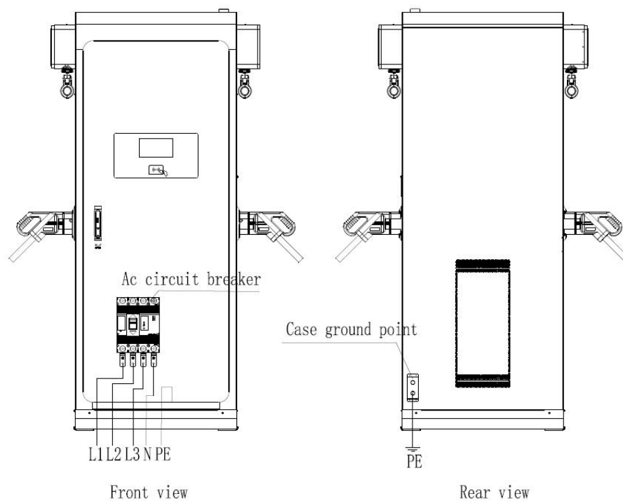
如图 3：充电桩接线图
