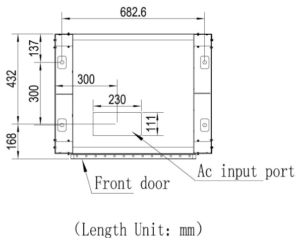
图 2：充电桩底座尺寸图
