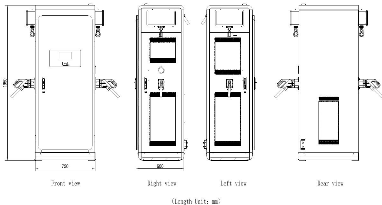
图 1：充电桩外形尺寸图
